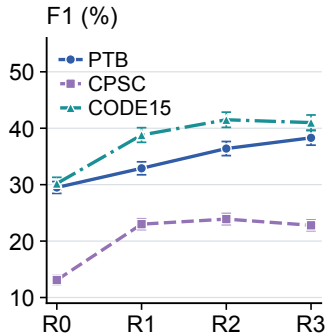
(b) Classification F1
